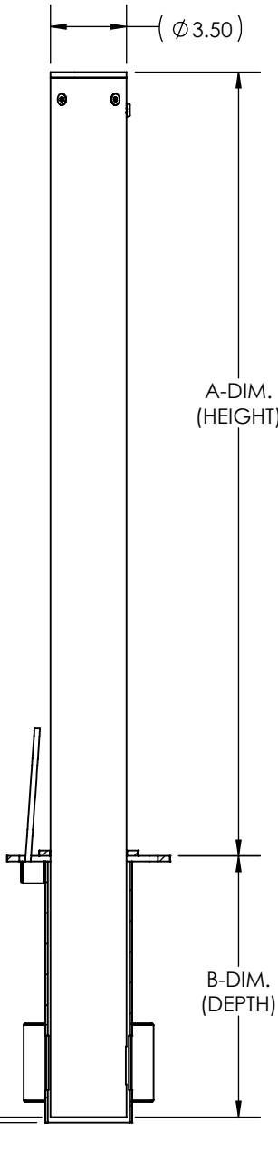
SECTION A-A
